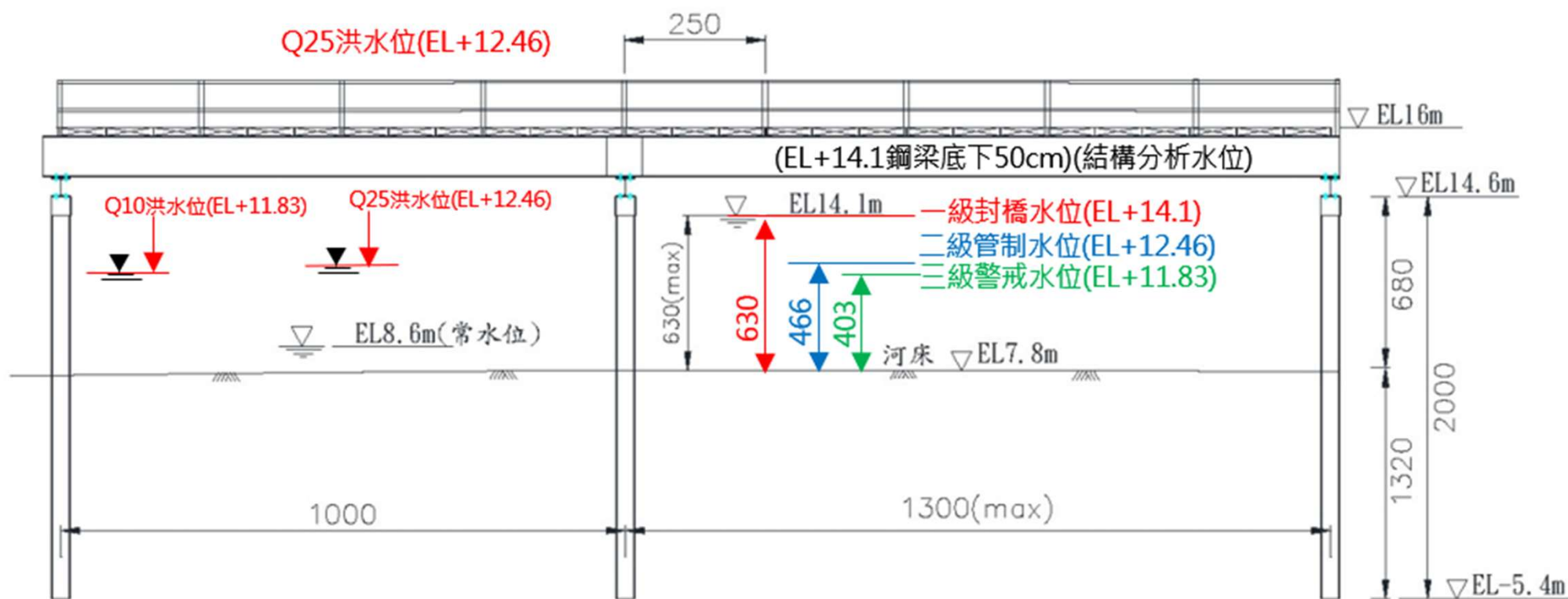
鋼便橋側視圖
