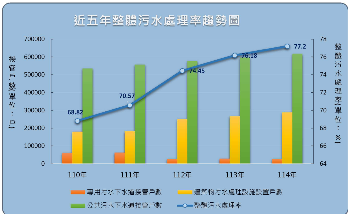
圖2：近五年整體污水處理率趨勢
