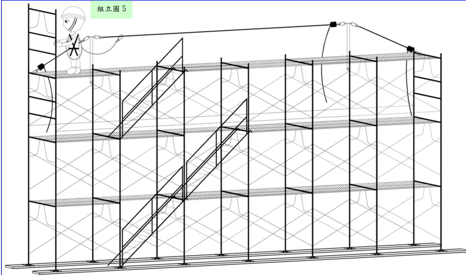
組立圖 5：(1)安全帶掛鉤鉤掛於水平母索，組立第 4 層施工架之立架（當層組立架而非由下層組立，避免造成立架飛落）。 (2)安全帶不得鉤掛於控索。(3)兩側之立架應裝設護欄（本圖為先裝設，亦可等第 4 層施工架組立完成再裝設）。
