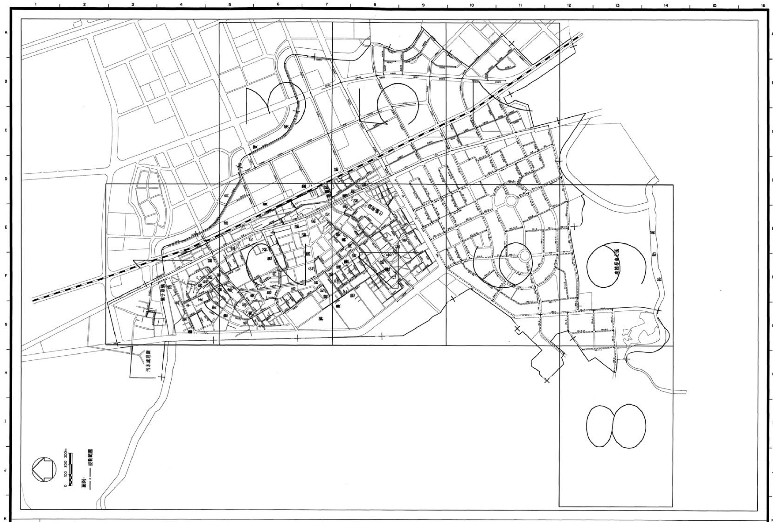
圖 4.3-4-4 橋頭地區污水下水道系統平面配置圖(索引圖)
