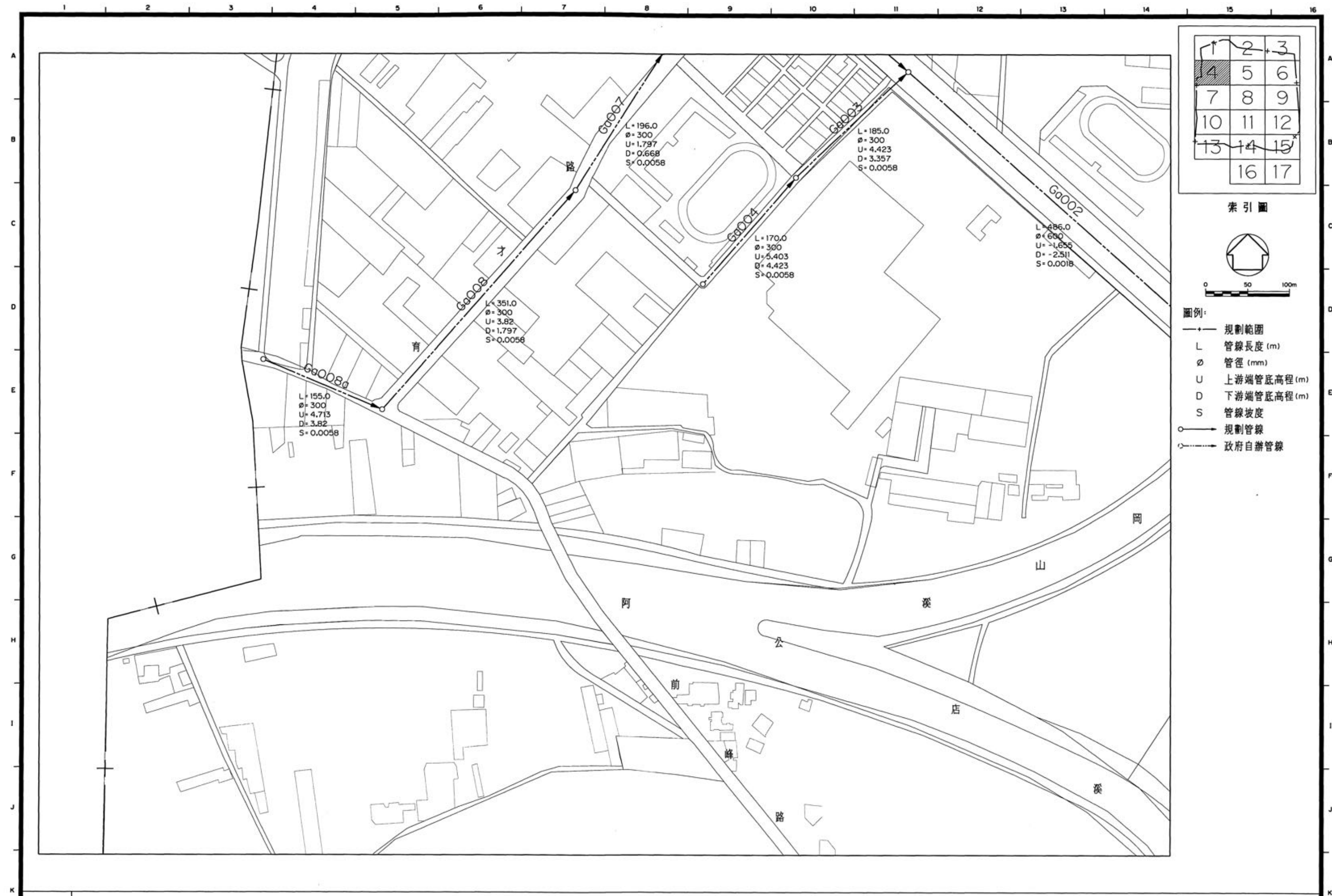
圖 4.5-4 岡山地區污水下水道系統平面配置圖 (4/17)
