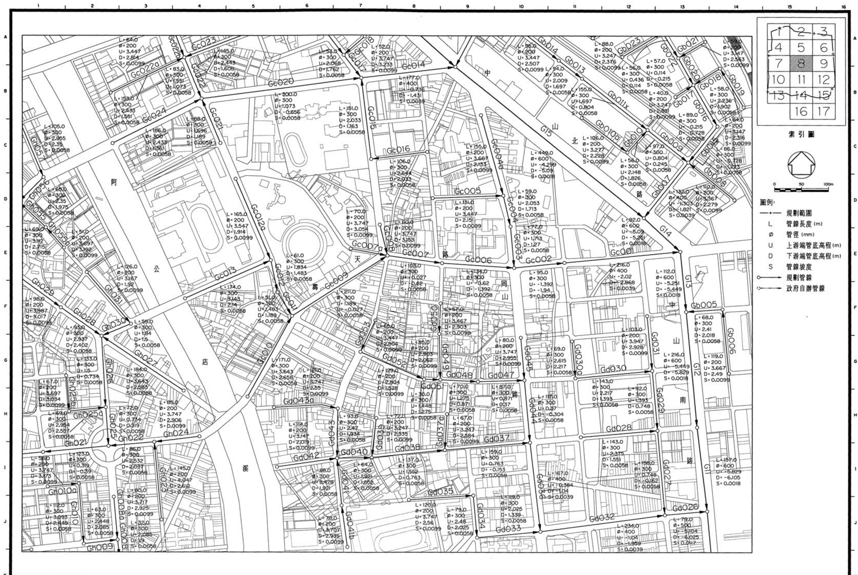
圖 4.5-4 岡山地區污水下水道系統平面配置圖 (8/17)
