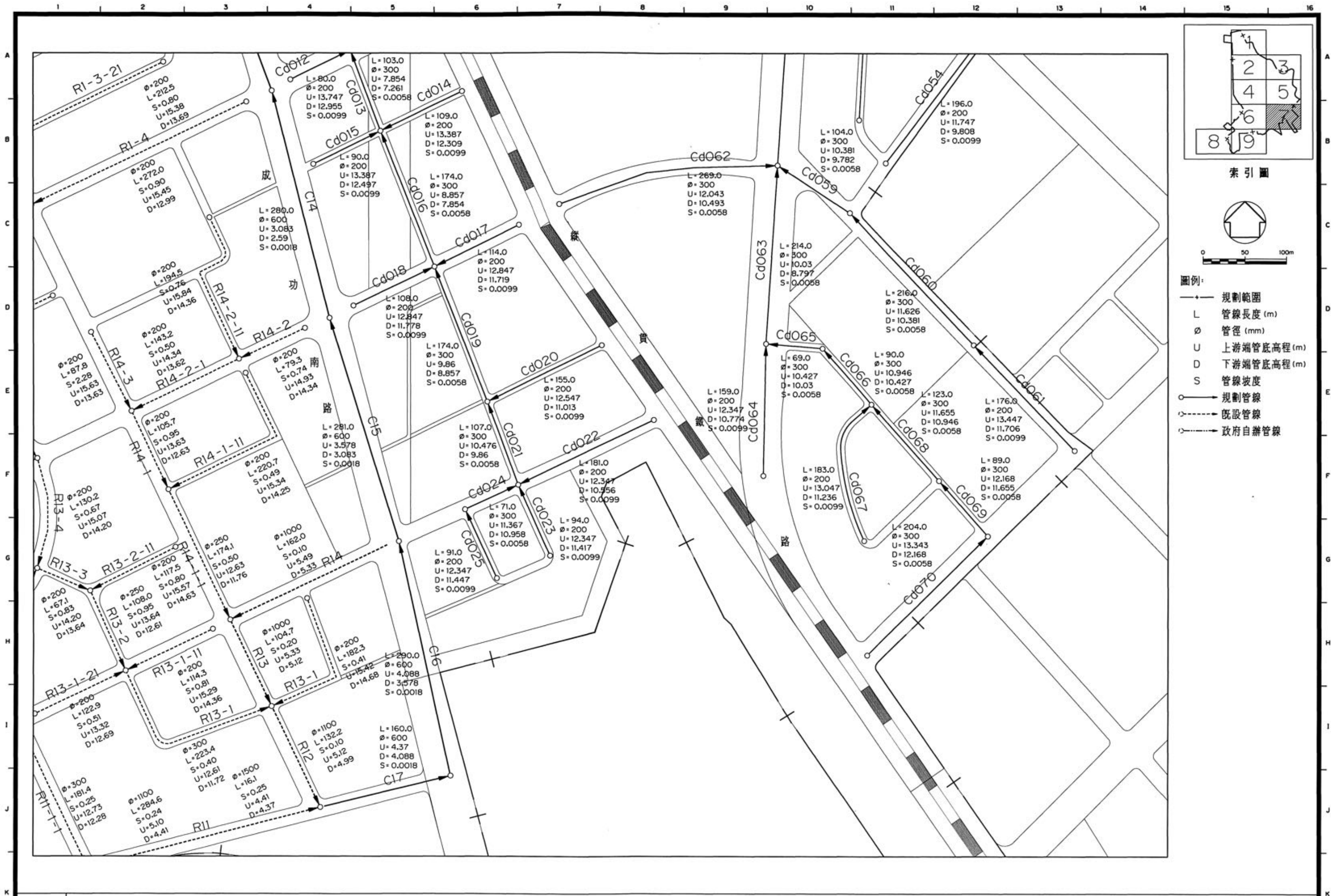
圖4.3.4-4 橋頭地區污水下水道系統平面配置圖(7/9)
