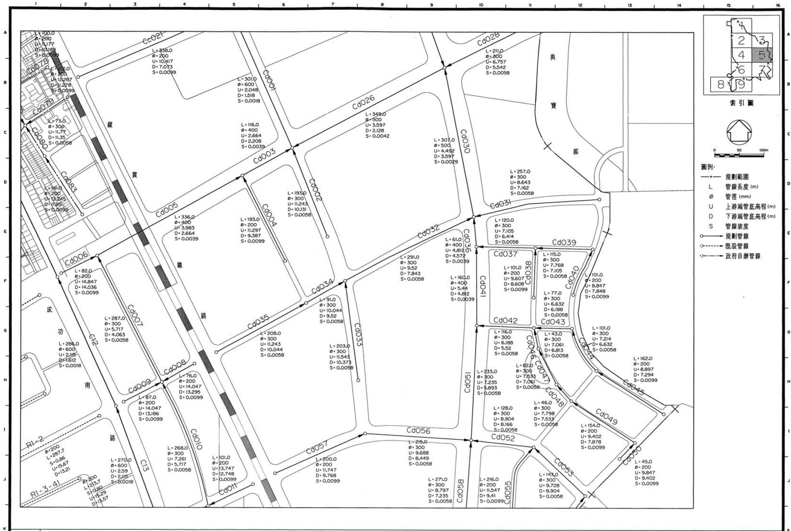
圖 4.3.4-4 橋頭地區污水下水道系統平面配置圖(5/9)
