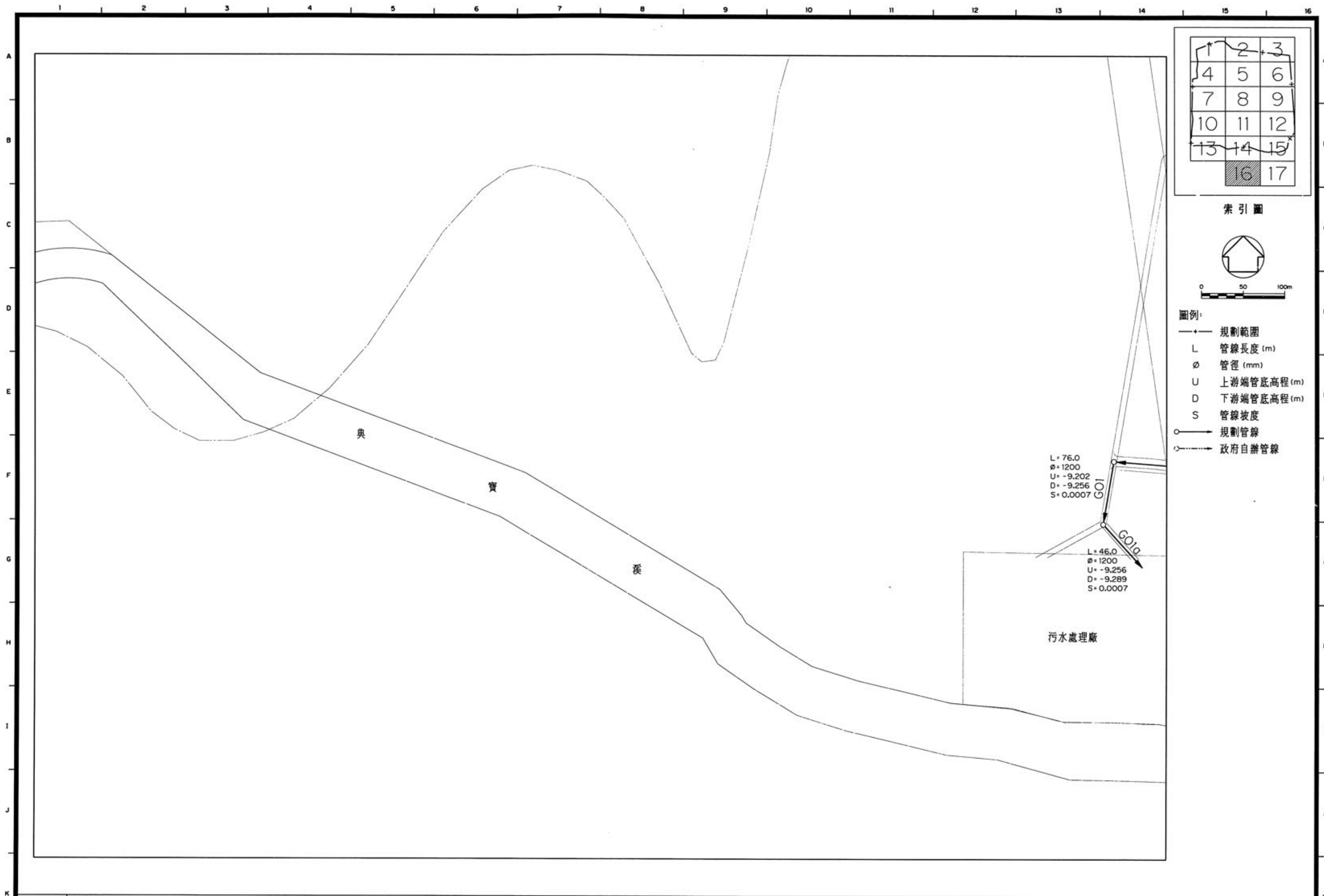
岡山地區污水下水道系統平面配置圖(16/17)
