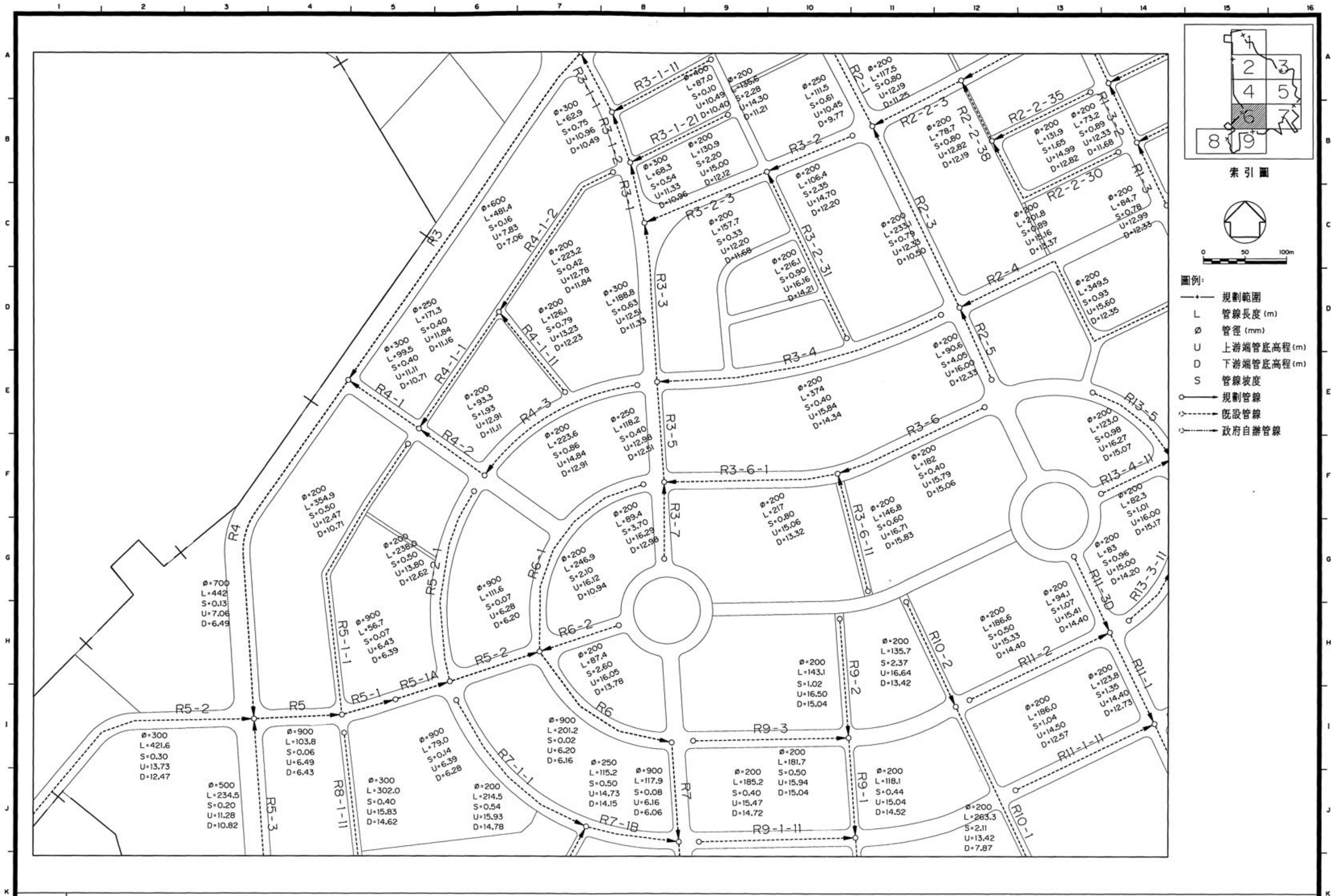
圖4.3.4-4 橋頭地區污水下水道系統平面配置圖(6/9)
