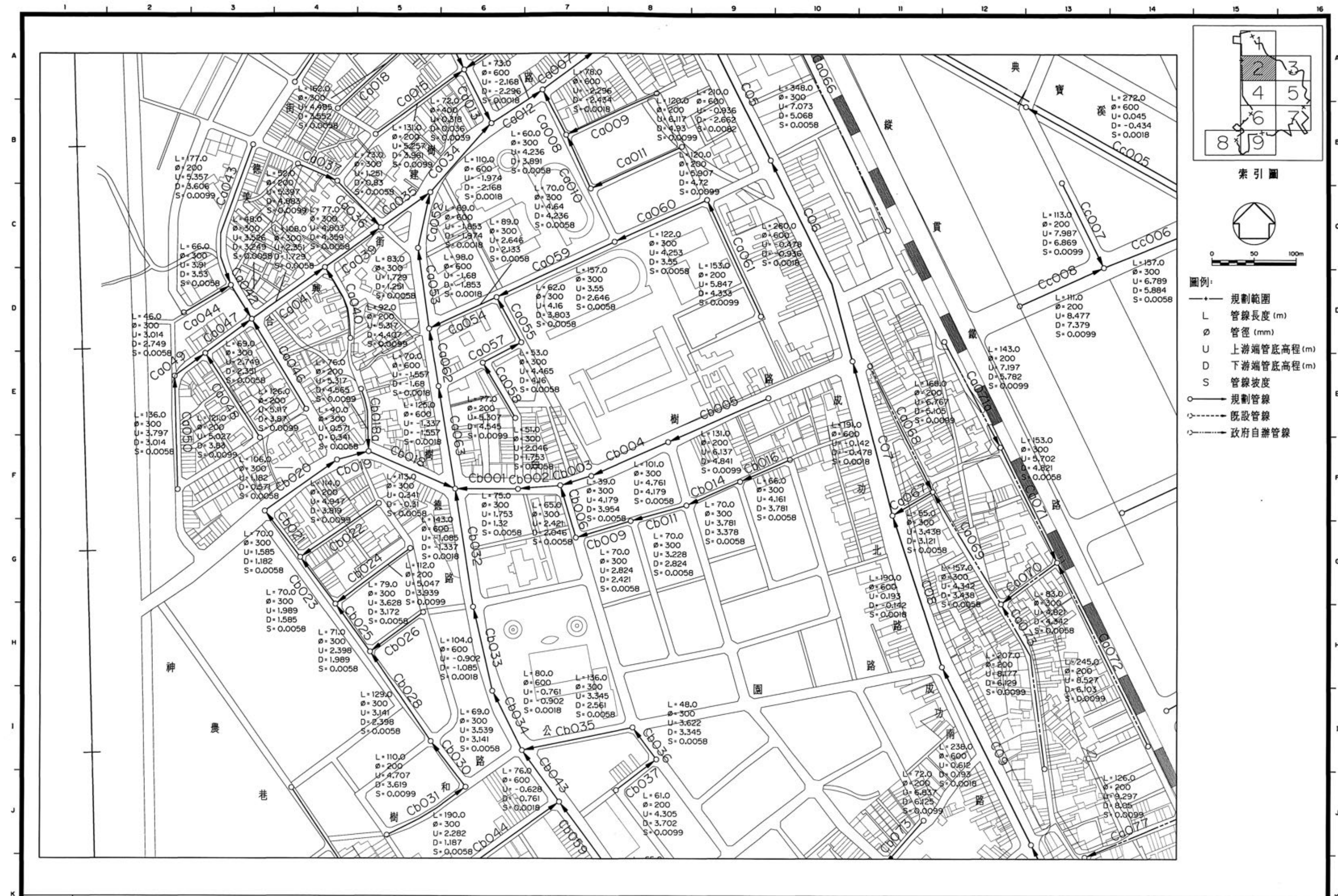
圖 4.3.4-4 橋頭地區污水下水道系統平面配置圖 (2/9)
