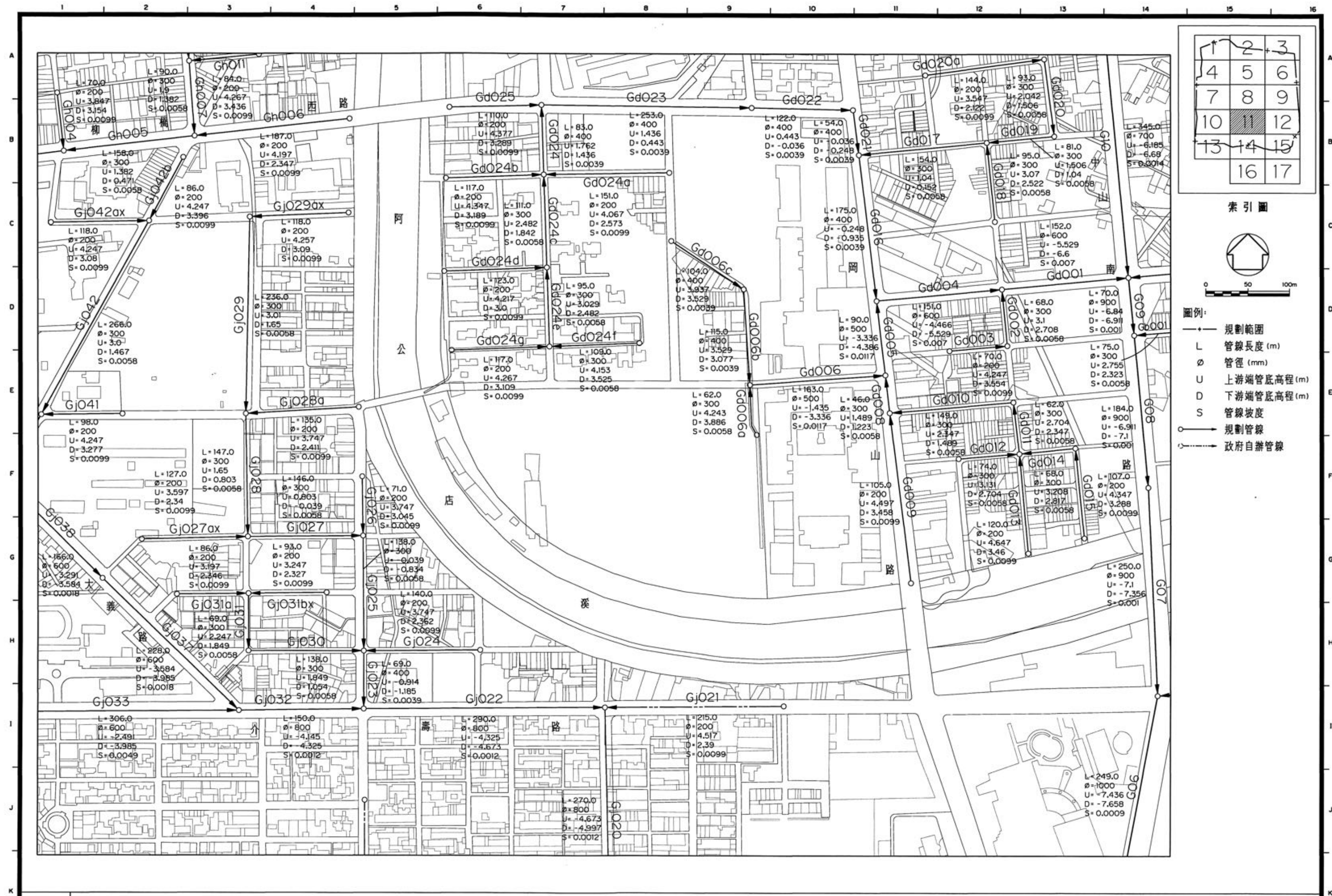
圖4.5-4 岡山地區污水下水道系統平面配置圖(11/17)
