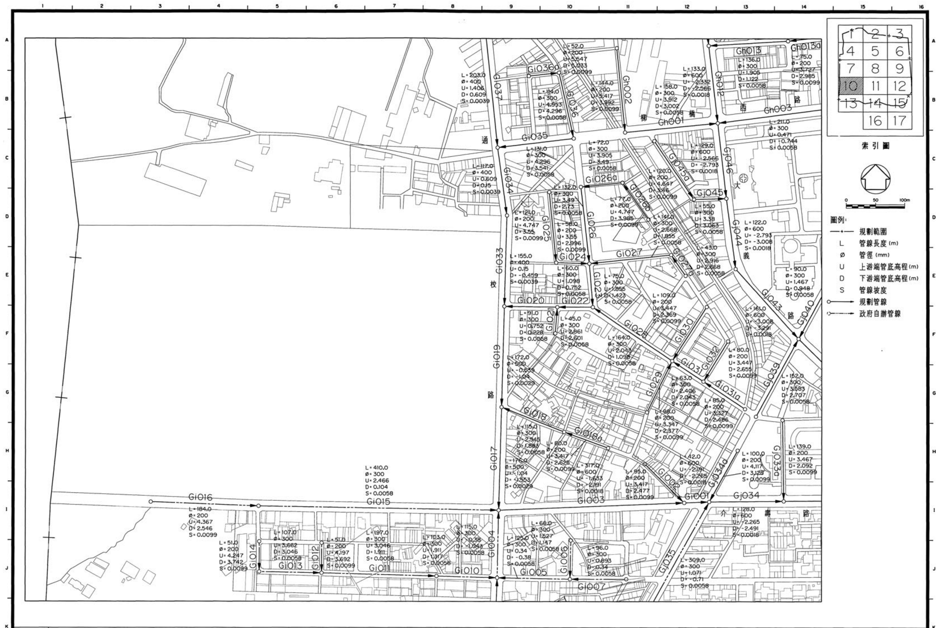
圖 4.5-4 岡山地區污水下水道系統平面配置圖 (10/17)
