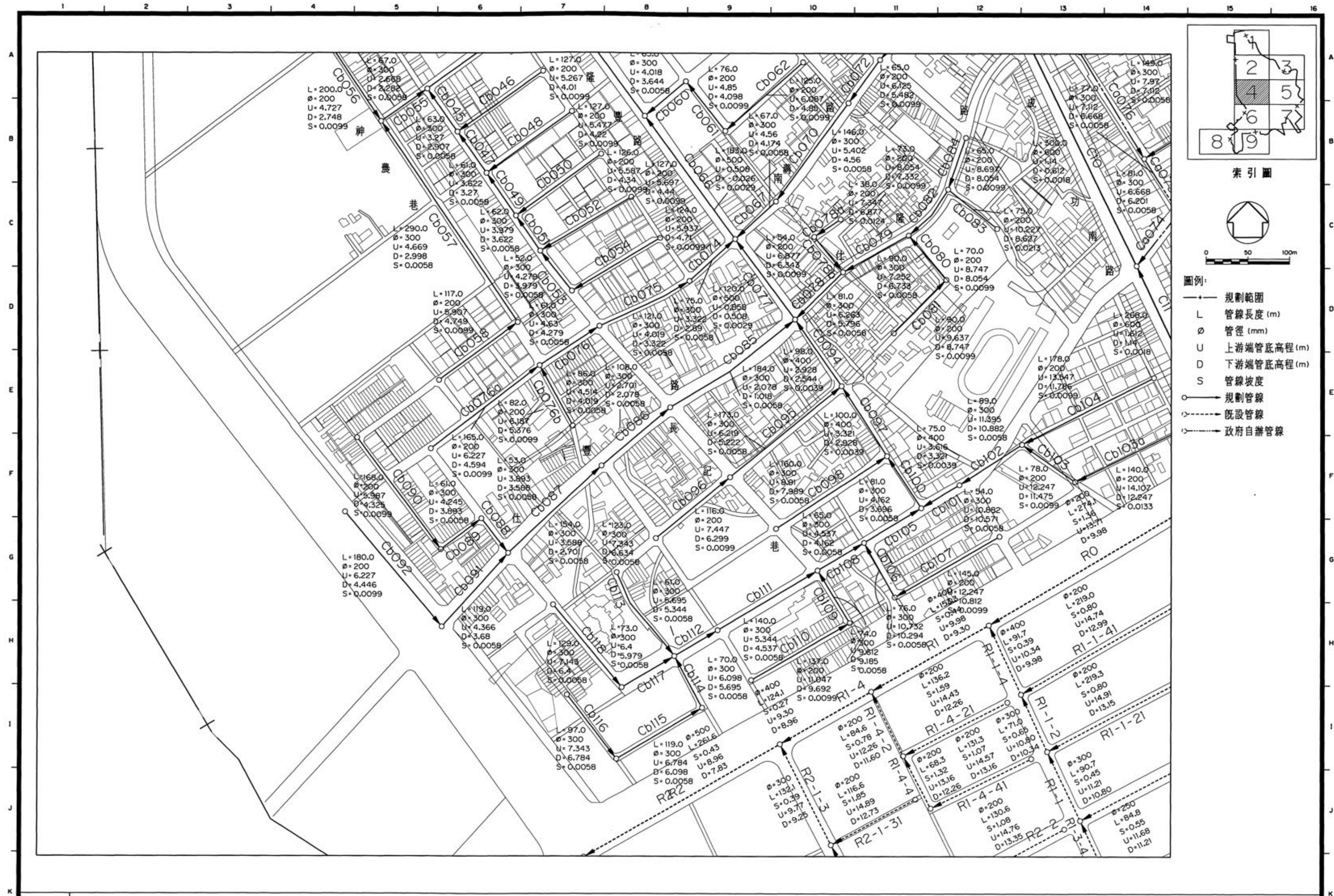
圖4.3.4-4 橋頭地區污水下水道系統平面配置圖(4/9)
