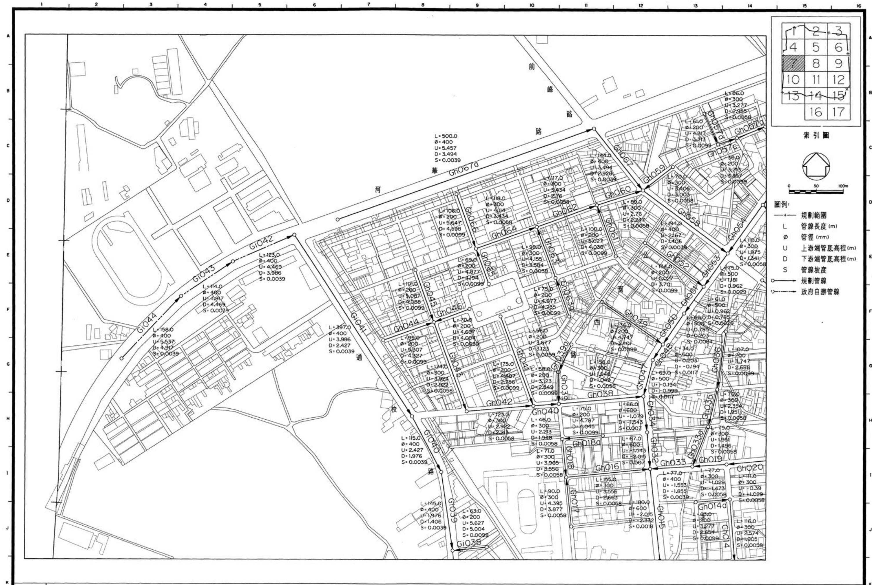
圖 4.5-4 岡山地區污水下水道系統平面配置圖(7/17)
