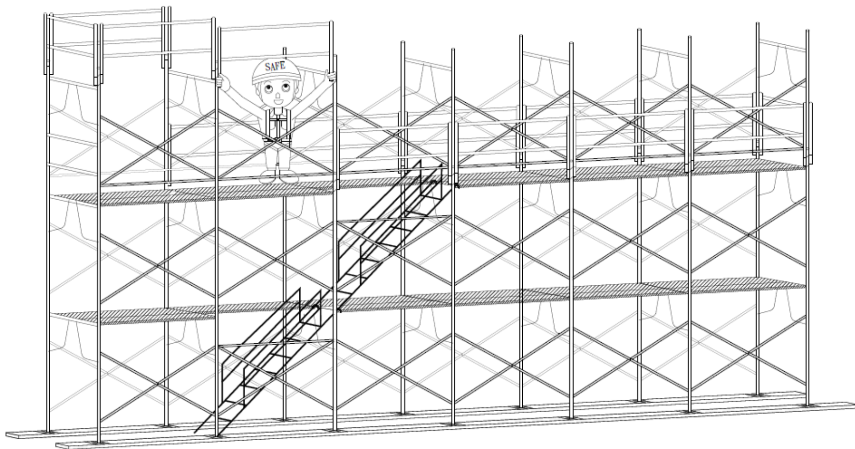
5. 下一階段先行扶手框組立示意圖
