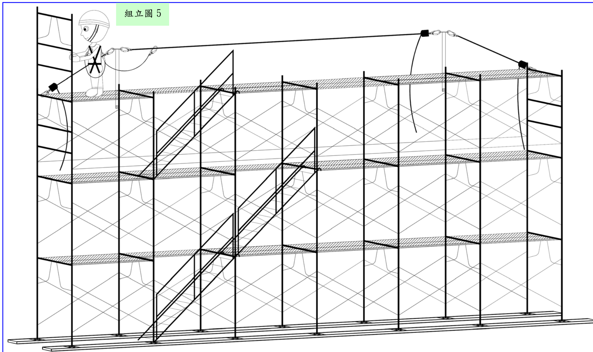
組立圖 5：(1)安全帶掛鉤鉤掛於水平母索，組立第 4 層施工架之立架（當層組立架而非由下層組立，避免造成立架飛落）。 (2)安全帶不得鉤掛於控索。(3)兩側之立架應裝設護欄（本圖為先裝設，亦可等第 4 層施工架組立完成再裝設）。
