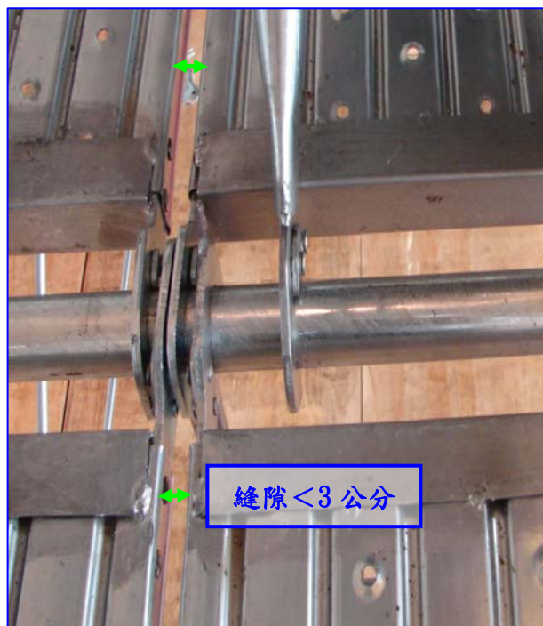
照片 3：工作台鋪滿密接之踏板，施工架踏板間之縫隙小於 3 公分。
